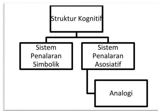
Gambar 1. Struktur Kognitif.
